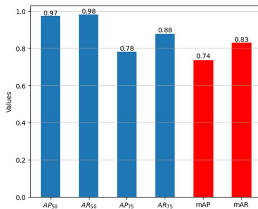
Figura 2.10: Risultati del sistema di rilevazione.
