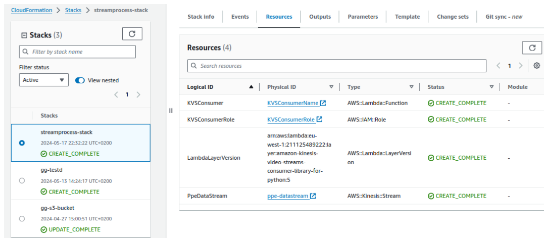
Figura 4.8: Stack set dell'infrastruttura di sistema.
