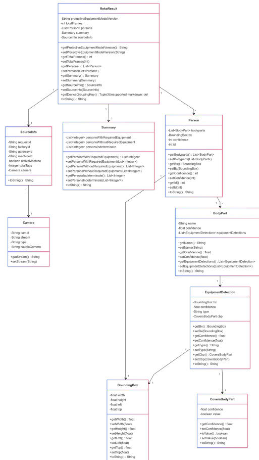
Figura 4.6: Diagramma modello dati.
