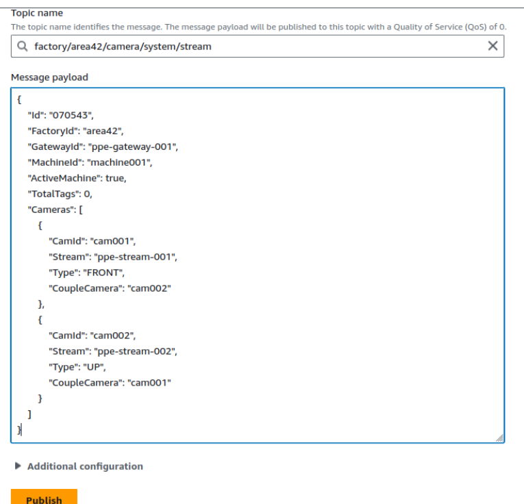
Figura 4.5: Pubblicazione messaggio MQTT su AWS IoT via console.
