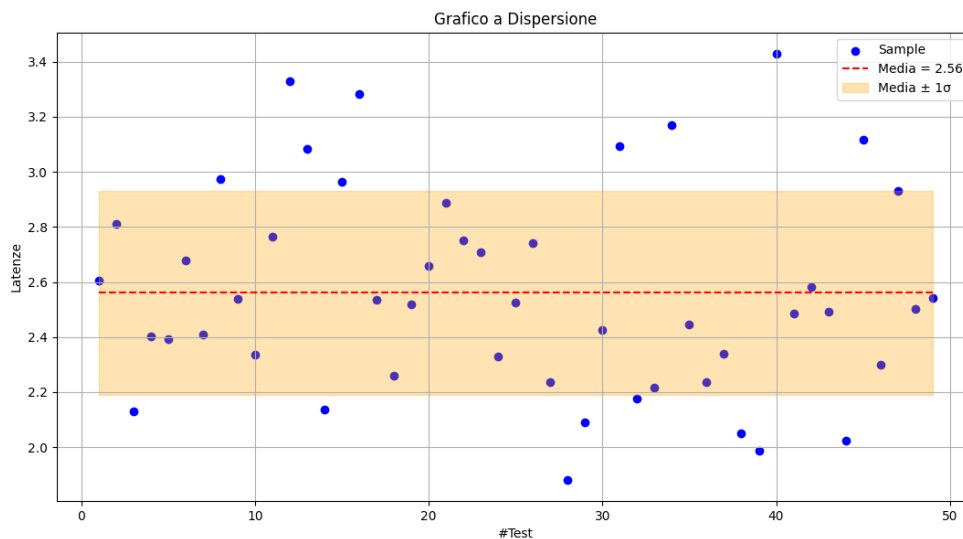
Figura 5.1: Latenza totale del sistema.
