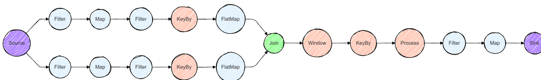
Figura 4.7: Dataflow logico del sistema.
