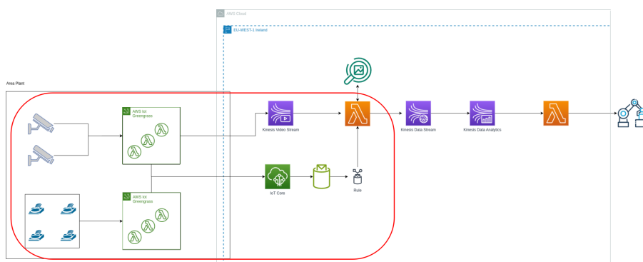
Figura 4.3: Sottosistema di ingestione e preprocessing.
