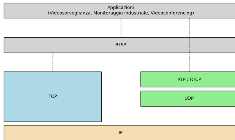
Figura 3.6: Stack di protocolli per lo streaming real-time.
