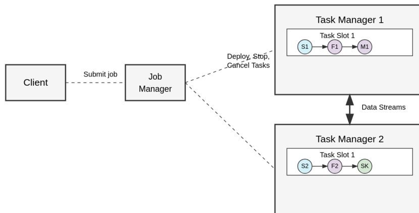
Figura 3.9: Esempio di funzionamento del runtime in Apache Flink.
