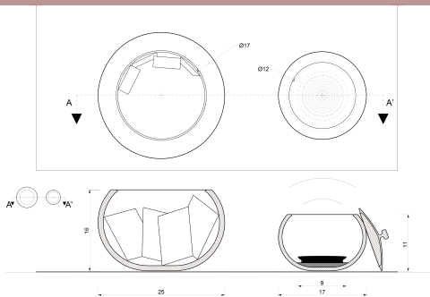
Viste ortogonali e sezione vasi Scala 1:5
