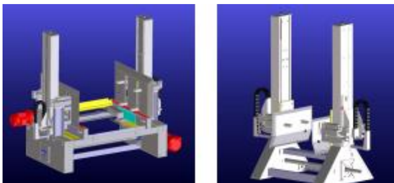
Fig 15. Stacker
