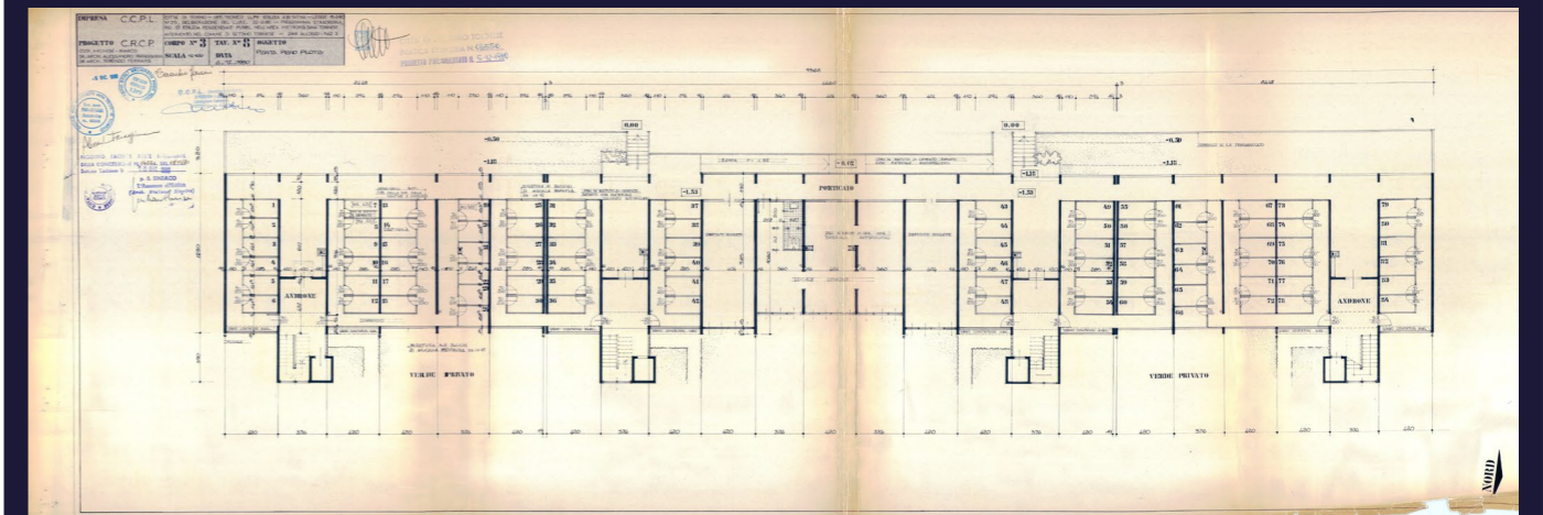
Fonte: Comune di Torino, Archivio edilizio, Ufficio tecnico II.pp. edilizia abitativa città di Torino, 1980, TAV 8, Pianta piano pilotis, Corpo 3
