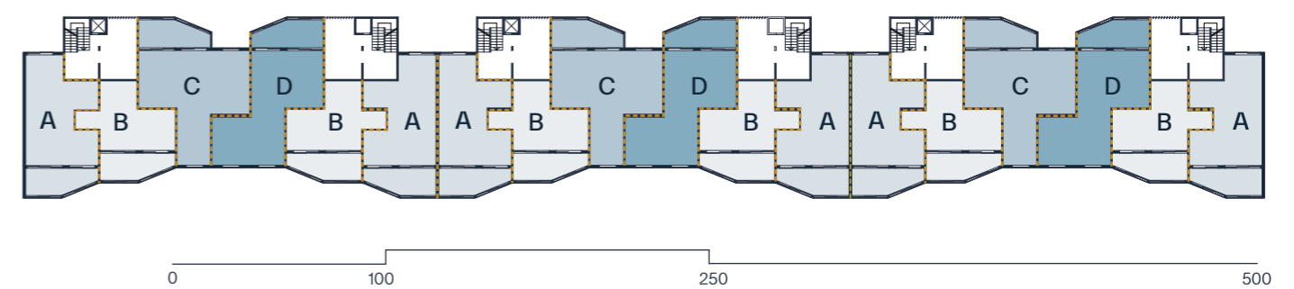
Fig. 2.41: Planimetria tipologie abitative - Stato di progetto
