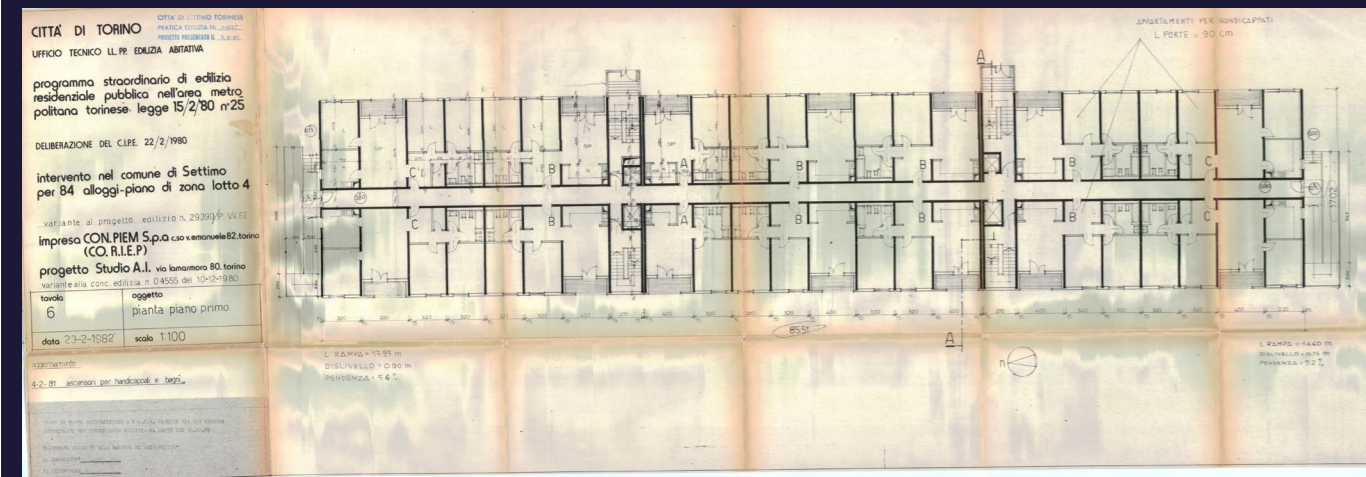
Fonte: Comune di Torino, Archivio edilizio, Ufficio tecnico ll.pp. edilizia abitativa città di Torino, 1980, TAV 6, Pianta piano primo.
