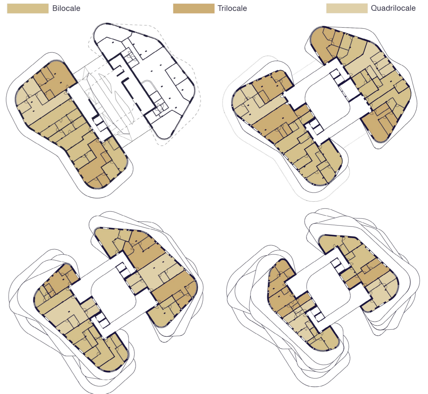
Fig. 2.59: Modelli planimetrici - Tipologia B
