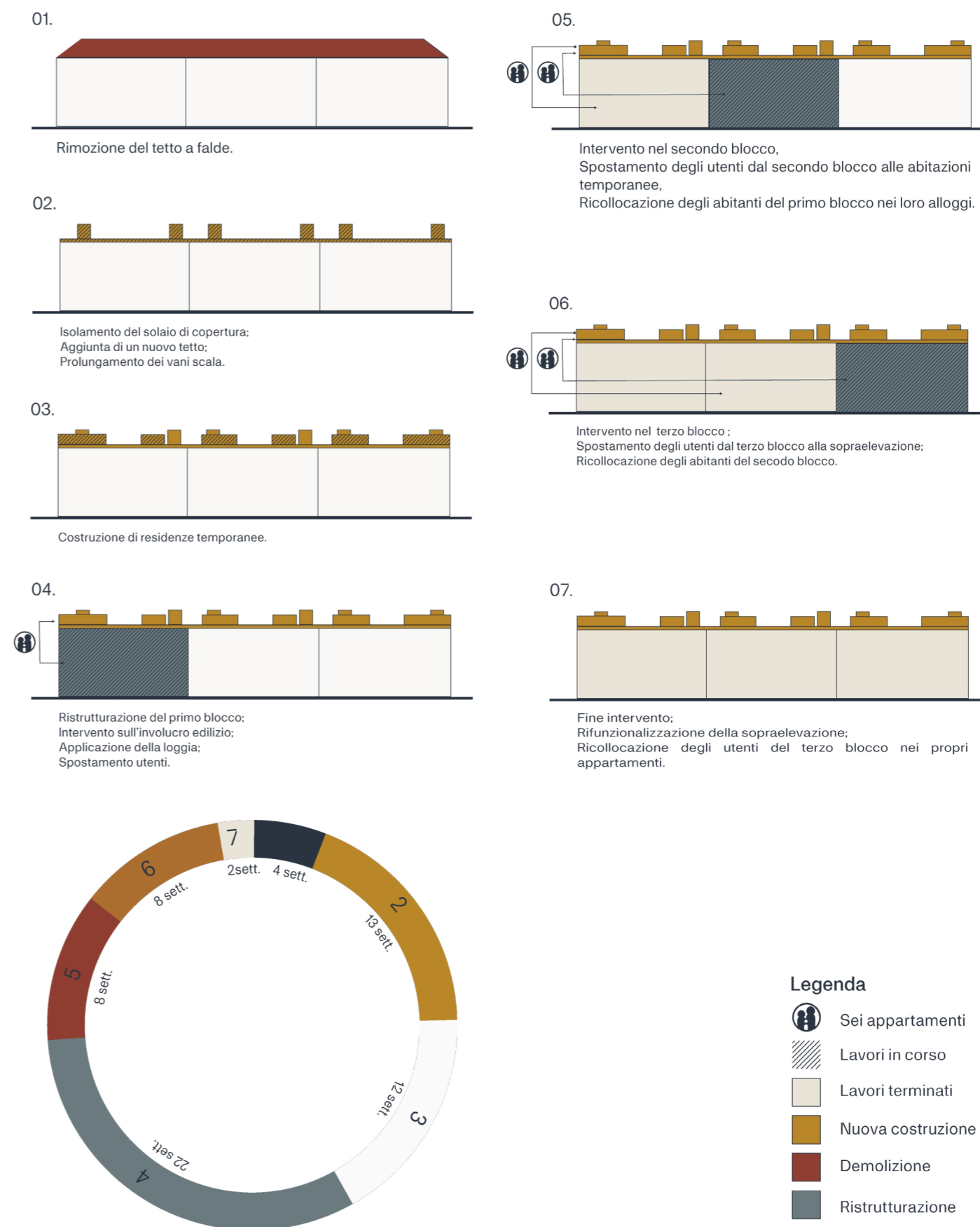
Fig. 2.27: Le fasi dei lavori e crono-programma
