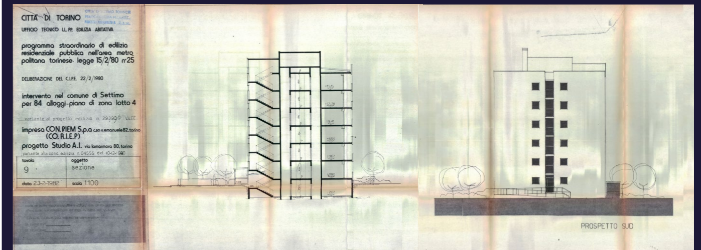
Fonte: Comune di Torino, Archivio edilizio, Ufficio tecnico ll.pp. edilizia abitativa città di Torino, 1980, TAV 9, Sezione.
