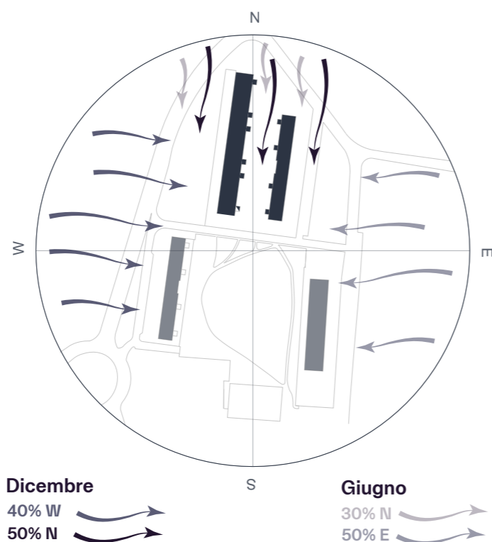
Fig. 2.5: Analisi della distribuzione e periodicità del vento nell'area di intervento
