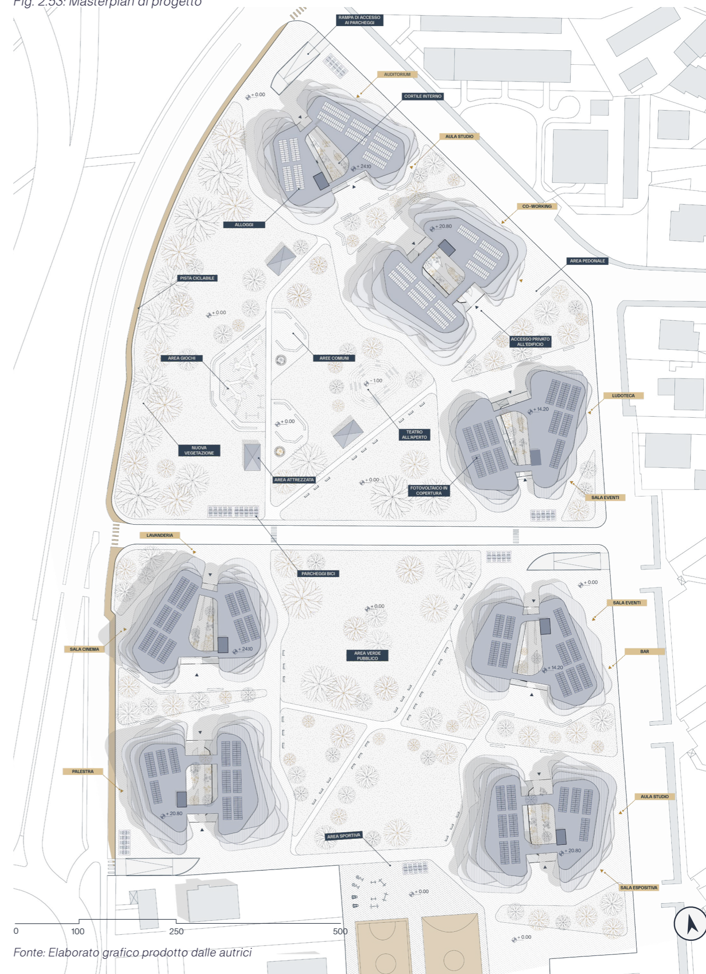
Fig. 2.53: Masterplan di progetto
