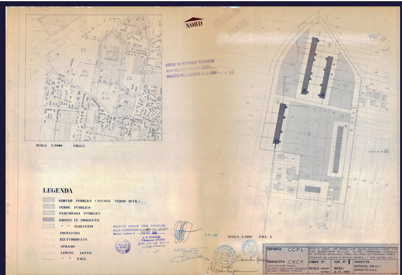
Fonte: Comune di Torino, Archivio edilizio, Ufficio tecnico II.p.p. edilizia abitativa città di Torino, 1980, TAV 1, Estratto PRG.
