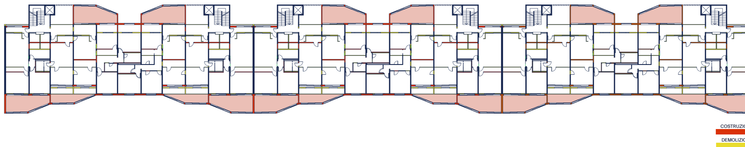
Fig. 2.33: Planimetria piano tipo - Progetto
