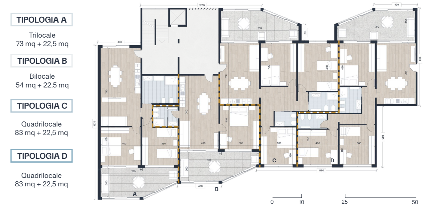
Fig. 2.41: Planimetria tipologie abitative - Stato di progetto
