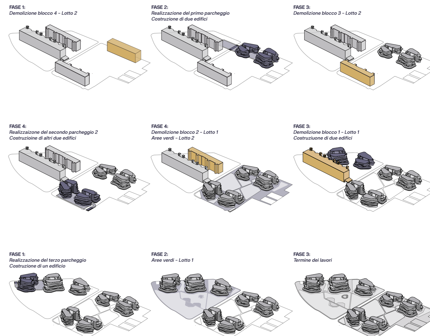
Fig. 2.55: Le fasi dei lavori
