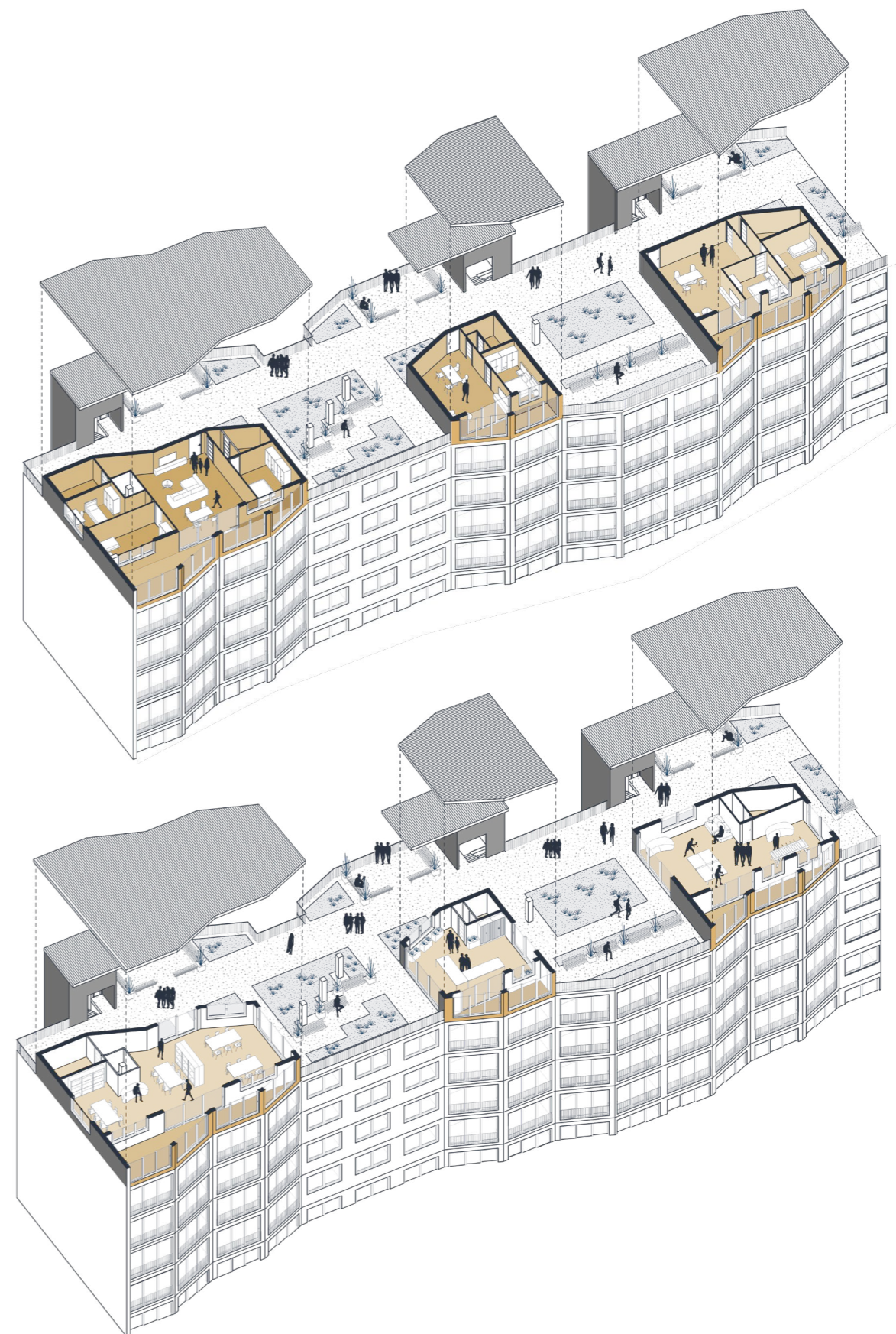
Fig. 2.44: Focus destinazione d'uso copertura
