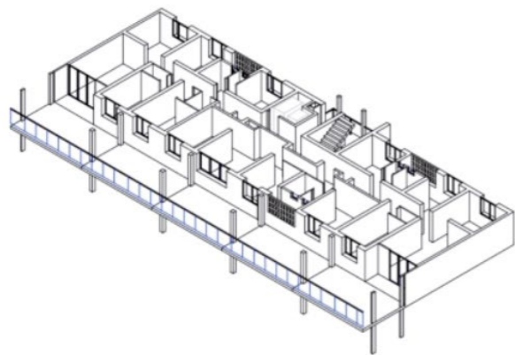
1 EXISTANT
