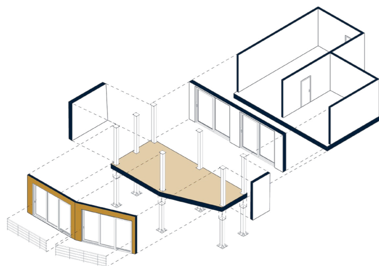
Fig.2.29: Schema composizione loggia
