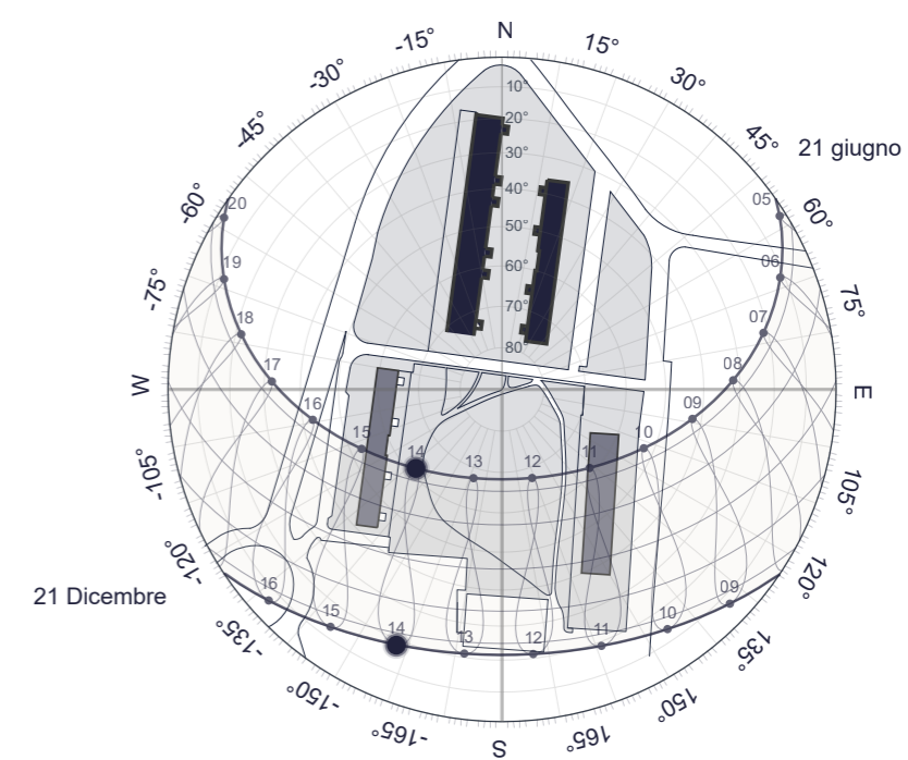
Fig. 2.7: Analisi dell'ombreggiamento applicata all'area di intervento
