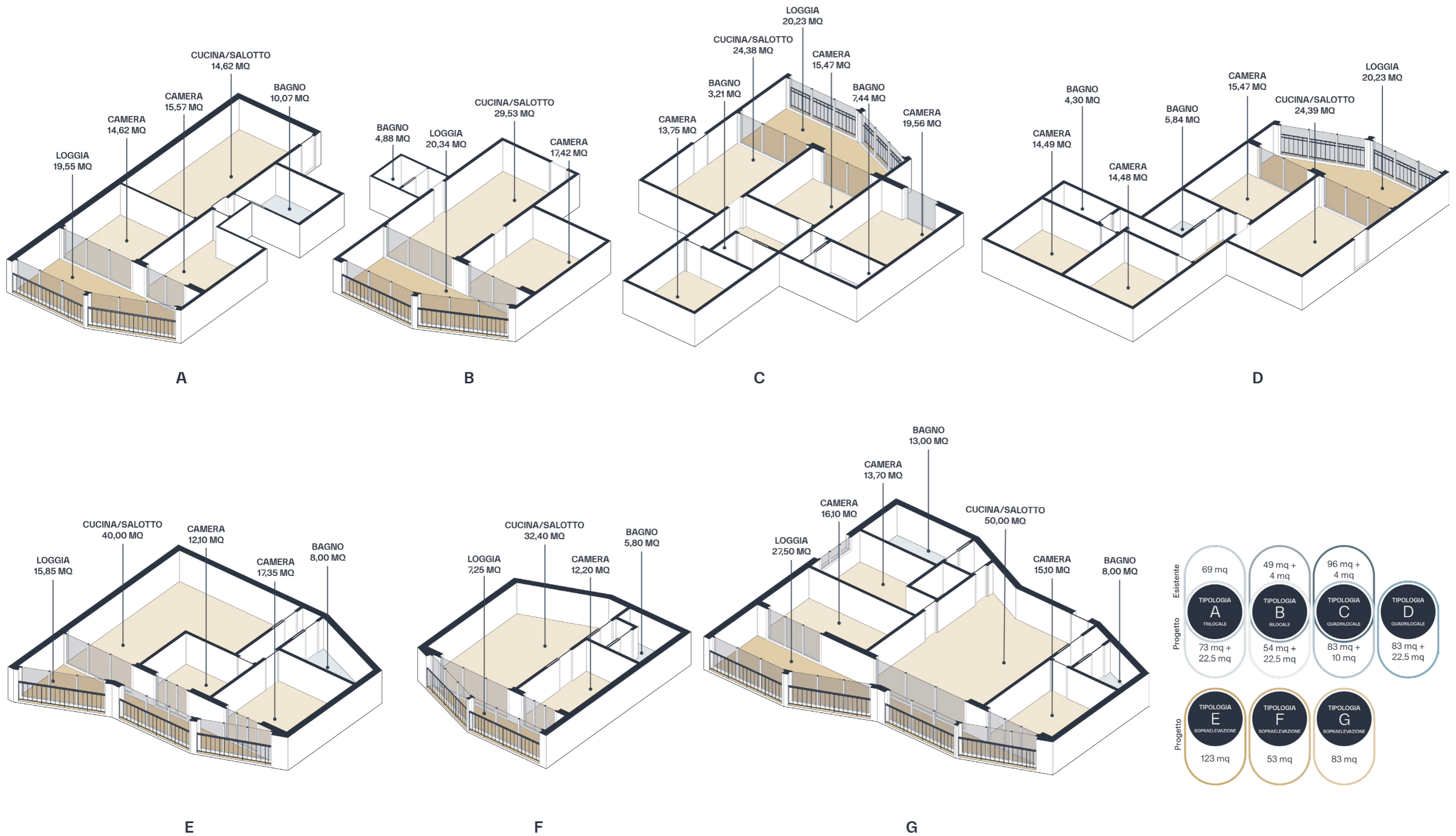
Fig. 2.45: Schema destinazioni d'uso ambienti interni per tipologia di alloggio
