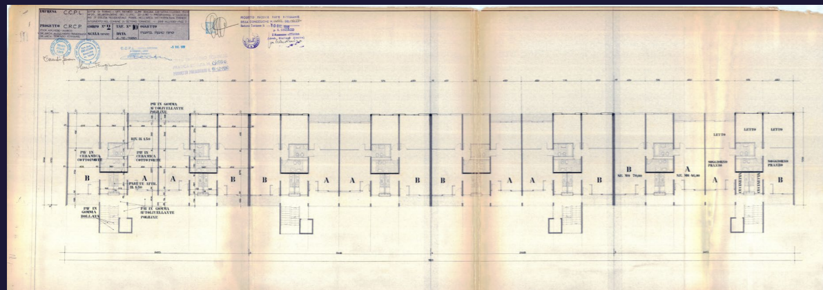
Fonte: Comune di Torino, Archivio edilizio, Ufficio tecnico II.pp. edilizia abitativa città di Torino, 1980, TAV 10, Pianta piano tipo, Corpo 2
