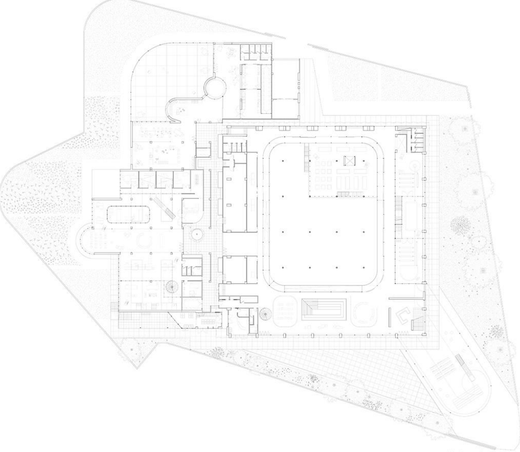
Planimetria generale
