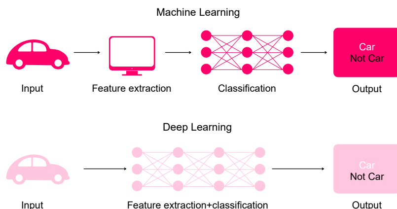
Figura 1.5: Analisi comparativa tra Machine Learning tradizionale e del Deep Learning. Grafico rielaborato.
