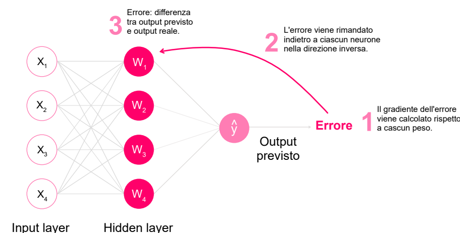
Figura 1.3: Rappresentazione schematica del processo di retropropagazione dell'errore (backpropagation) in una rete neurale multistrato (MLP). Grafico rielaborato.
