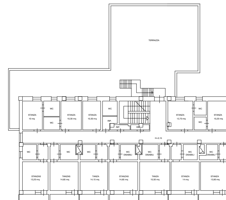
Pianta piano terzo
