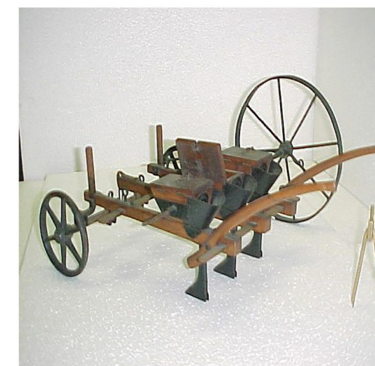
| Foto a destra: Seminatrice sottosuperficiale a 3 file Modello conservato presso il Laboratorio di agraria dell'ITCG di Vercelli, da www.roberto-crosio.net/1_vercellese/cavour_macchine_concimi.htm
