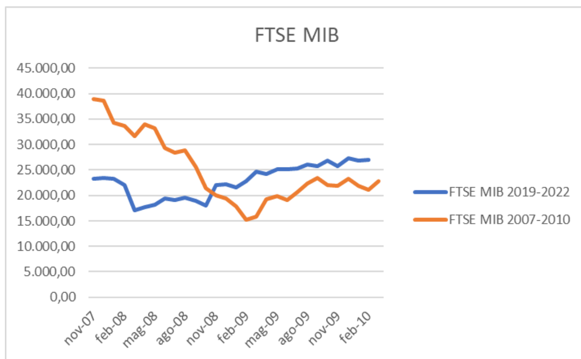
Figura 14 Andamento FTSE MIB
